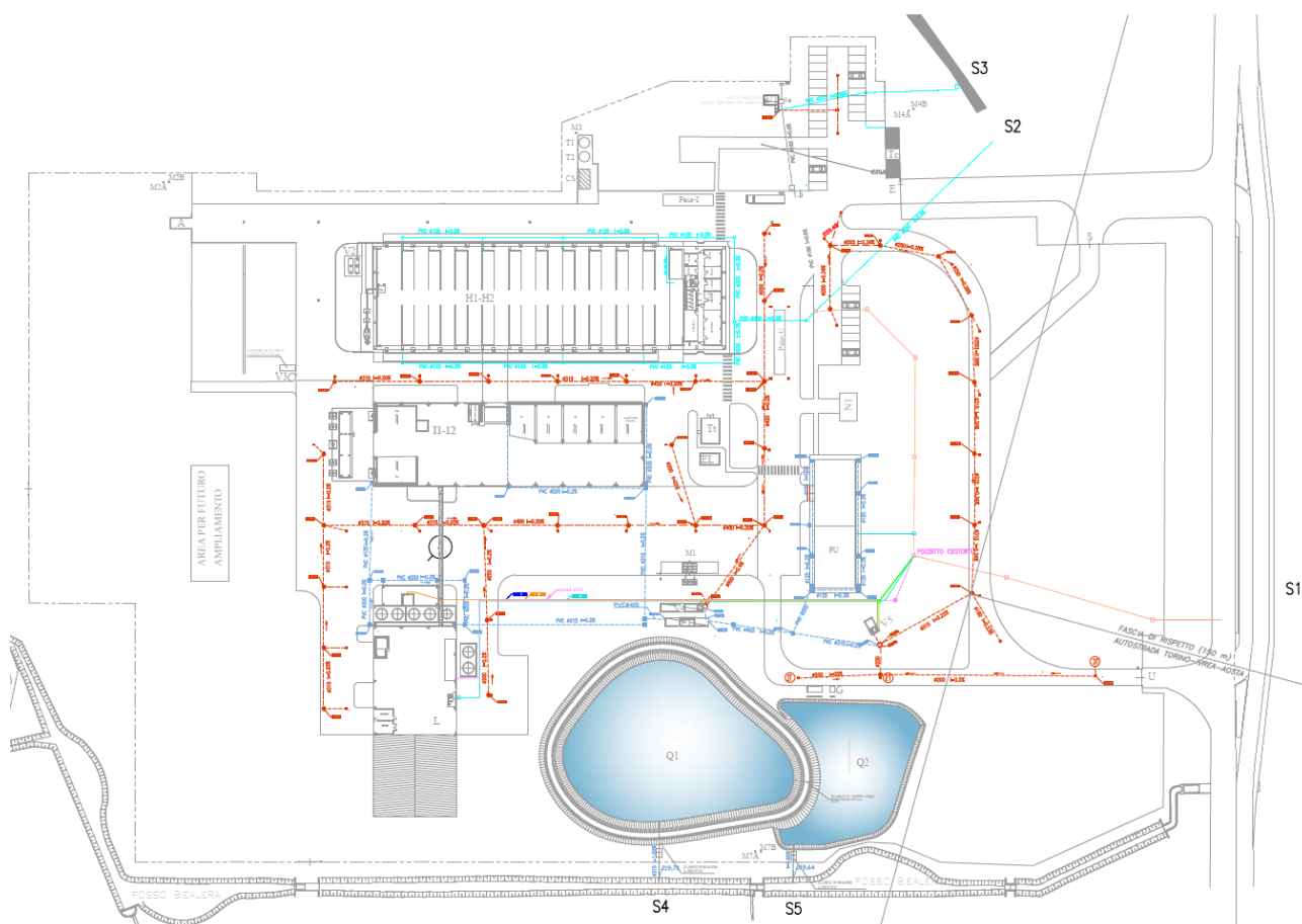
Figura 12 – Planimetria scarichi
